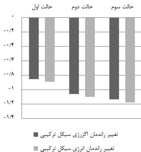
شکل ۹) تأثیر سیستم احتراق اضافه بر بازده اگزورزی و انرژی سیکل ترکیبی
