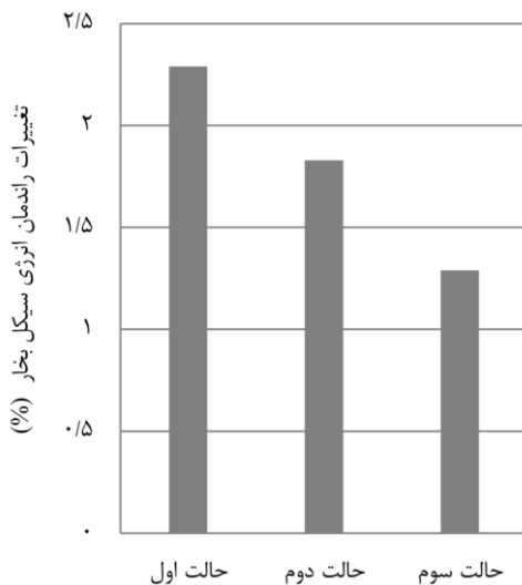
شکل ۵) تأثیر سیستم احتراق اضافه بر بازده آگزردی سیکل بخار
