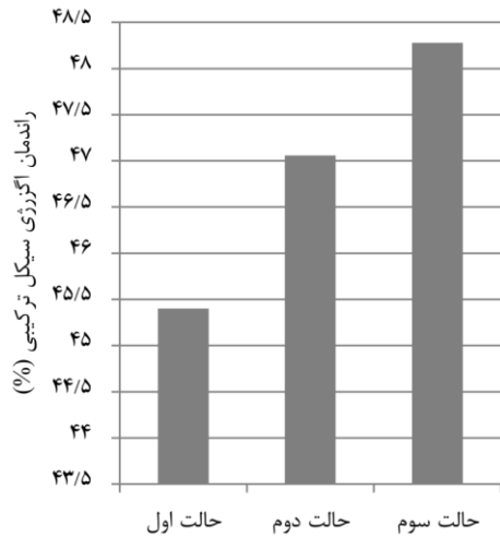
شکل ۸) بازده اگزورزی سیکل ترکیبی در حالات مختلف بهره‌برداری بدون استفاده از سیستم احتراق اضافه
