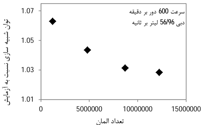
شکل 3 توان خروجی توربین و نسبت مقدار عددی به تجربی به‌ازای شبکه‌های محاسباتی مختلف برای توربین با پره‌های باز و مدل آشفتگی تنش برشی انتقالی
