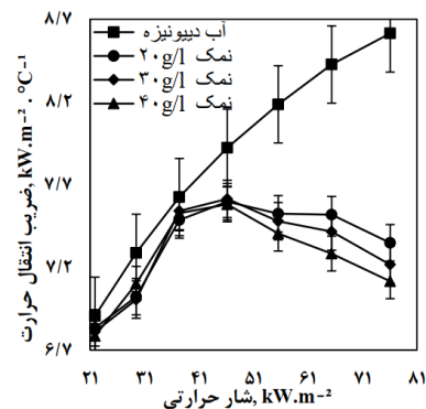
شکل ۳) مقایسه ی تغییرات غلظت بر ضریب انتقال حرارت
