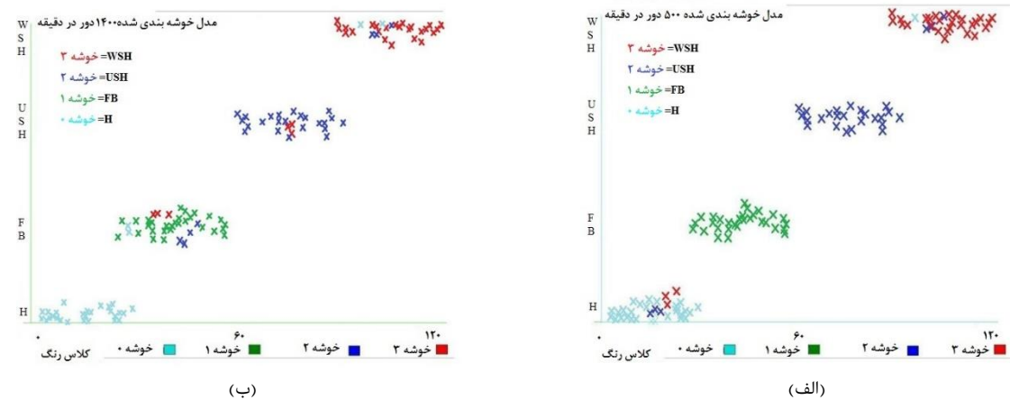
شکل ۷) (الف) پراکنندگی نمونه‌ها در خوشه‌بندی مربوط به ۵۰۰ دور در دقیقه. (ب) پراکنندگی نمونه‌ها در خوشه‌بندی مربوط به ۱۴۰۰ دور در دقیقه
