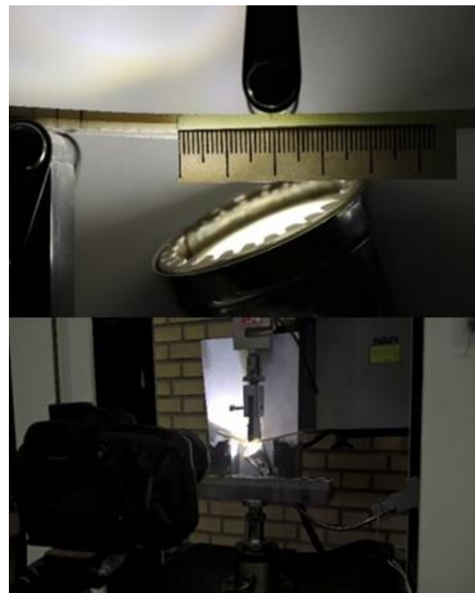
شکل ۴ تجهیزات آزمایشگاهی و تنظیم دستگاه جهت انجام آزمایش شکست
