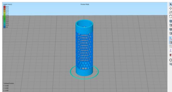
شکل ۵) نمایی از آماده‌سازی استنت در برنامه سیمپلی‌فای‌تری‌دی
