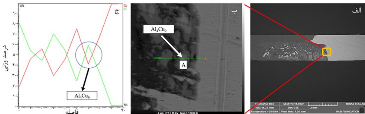
شکل ۱۰) الف) تصویر SEM مقطع TD-ND نمونه ۳۰ درصد نورد، (ب) تصویر SEM مقطع TD-ND نمونه ۳۰ درصد نورد در مرز جوش با بزرگنمایی بالاتر و (ج) نمودار تغییرات درصد وزنی عناصر آلومینیوم و مس ناشی از آنالیز عنصری EDS متناظر با تصویر SEM
