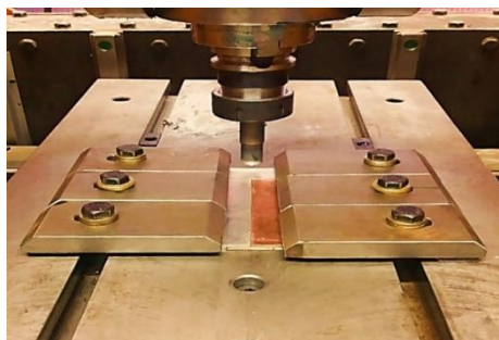
شکل ۲) دستگاه جوشکاری اصطکاکی-اغتشاشی و انجام جوشکاری با ابزار فولادی
