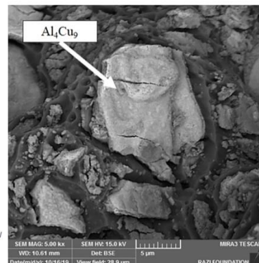
شکل ۱۲ تصاویر BSE و آنالیز EDX مربوط به سطح شکست نمونه ۳۰ درصد نورد از سمت آلومینیوم
