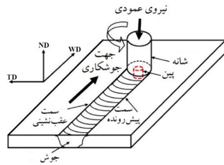
شکل ۱) شماتیک روش جوشکاری اصطکاکی-اغتشاشی (FSW) و دستگاه مختصات واقع بر نمونه جهت جوشکاری: WD، جهت عرضی: TD و جهت عمودی: ND
