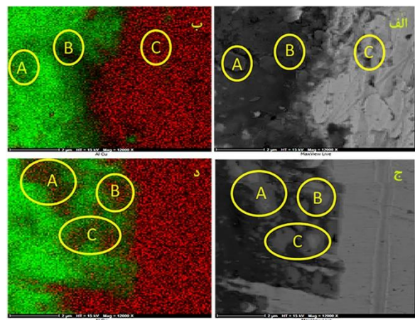
شکل ۷) تصاویر SEM و نقشه EDS متناظر با آن برای نمونه های الف) و ب) صفر درصد نورد و ج) و د) ۳۰ درصد نورد
