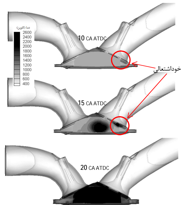
شکل 11 شکل شعله در مقطع زده شده با 3/25 سانتی متر فاصله از مرکز محافظه احتراق (نزدیک سوپاپ دود)
