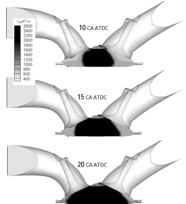
شکل 10 شکل شعله در مقطع زده شده از مرکز محافظه احتراق (محل شمع)
