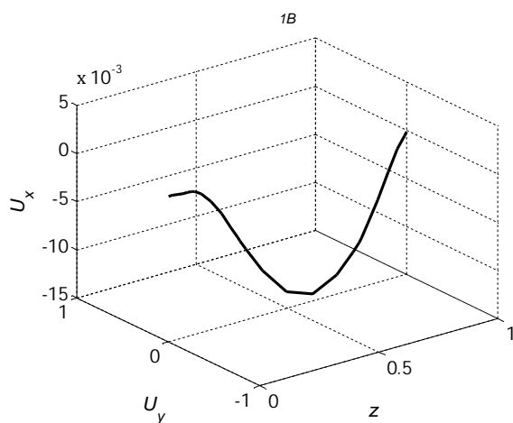
شکل 5-ب شکل مود متناظر با فرکانس اول پسر به ازای \gamma=200
