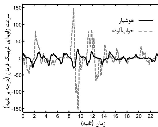
شکل 16 نمودار سرعت زاویه‌ای غریبک فرمان برای راننده شماره 5 در دو حالت هوشیار و خواب‌آلوده
