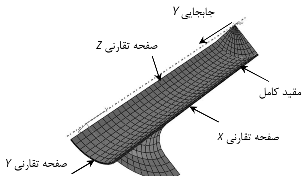
شکل 6 مدل شبیه‌سازی اجزای قالب
