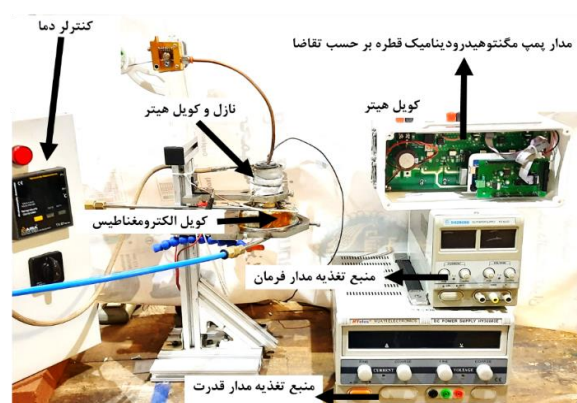
شکل ۲) نمای کلی از دستگاه طراحی شده
