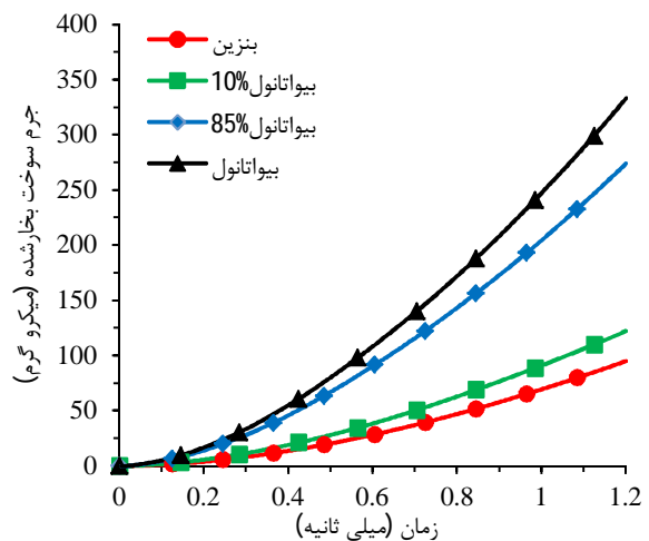
شکل 16 مقایسه جرم سوخت بخار شده در حین تزریق با ثابت ماندن انرژی سوخت تزریق شده و مدت زمان پاشش
