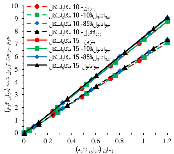
شکل 10 مقایسه‌ی جرم سوخت تزریق شده با افزایش فشار تزریق از 10 مگاپاسکال به 15 مگاپاسکال
