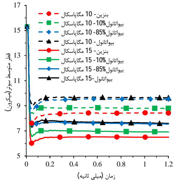
شکل 15 مقایسه قطر متوسط سوتر سوخت های مورد بررسی با افزایش فشار تزریق 10 مگاپاسکال به 15 مگاپاسکال
