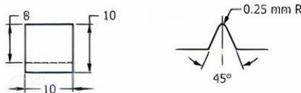
شکل ۱) اندازه نمونه‌ی استاندارد شارپی مورد استفاده در این تحقیق [21]
