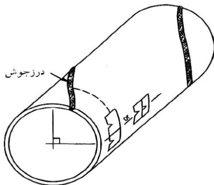
شکل ۲) موقعیت استخراج نمونه‌های استاندارد شارپی از لوله API X70 با درز جوش ماریپیج [22]
