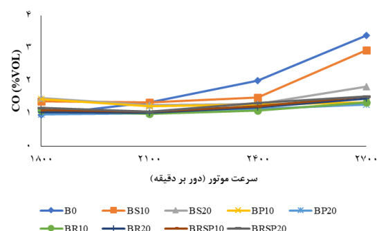
شکل ۱۰ تغییرات آلایندہ CO موتور با سرعت‌های مختلف برای سوخت‌های آزمایش شده
