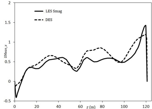
شکل 15 مقایسه سرعت‌های متوسط میانگین در جهت X در حد فاصل بین ضلع شمالی دانشکده فنی و ضلع جنوبی دانشکده علوم پایه
