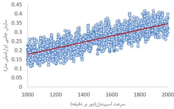
شکل ۸) تأثیر سرعت اسپیندل بر سایش ابزار
