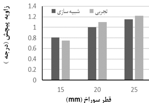
شکل ۶) مقایسه نتایج زاویه پیچش مربوط به آزمایش تجربی و شبیه سازی
