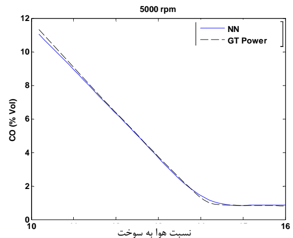
شکل 24 مقایسه تأثیر تغییرات نسبت هوا به سوخت بر آلاینده CO در مدل شبکه عصبی با مدل جی تی پاور، در سه دور نمونه ای 5000، 3500 و 2000
