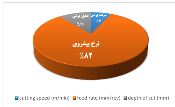
شکل ۷) درصد تأثیر پارامترهای مختلف بر زبری سطح
