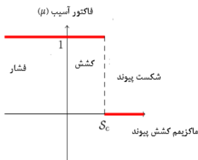
(ب): ارتباط فاکتور آسیب با تغییر طول نسبی بردار پیوند میان نقاط مادی
