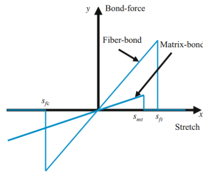
شکل ۷) ارتباط بین نیروی موجد در بردار پیوند در جهت الیاف و ماده زمینه با تغییر طول بردار پیوند
