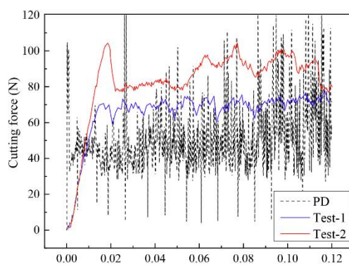
زاویه الیاف 90°
