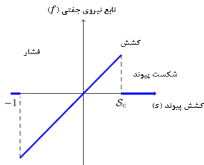
(الف): ارتباط تابع نیروی جفتی با تغییر طول نسبی بردار پیوند میان نقاط مادی شکل ۴- نمایش ارتباط تابع نیروی جفتی و فاکتور آسیب با تغییر طول نسبی بردار پیوند میان نقاط مادی
