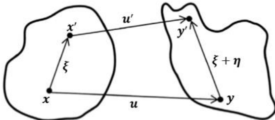
شکل ۲- مفهوم تغییرشکل پیکربندی مرجع در تئوری پری دینامیک
