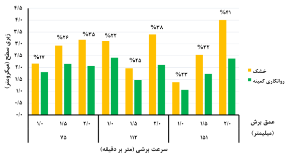
شکل ۲) نمودار زبری سطح بر اساس عمق برش، حالت روانکاری و سرعت برشی
