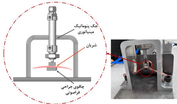
شکل ۳) نحوه عملکرد چاقوی جراحی فراصوتی در دوخت سرخرگ کاروتید گوسفند
