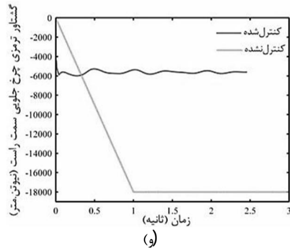
شکل 4 نتایج شبیه‌سازی در حالت با و بدون کنترل برای چرخ جلو راست: الف) لغزش، ب) سرعت چرخ و خودرو در حالت کنترل شده، ب) سرعت چرخ و خودرو در حالت کنترل نشده، ج) لغزش چرخ، د) نیروی ترمزی، و) گشتاور ترمزی
