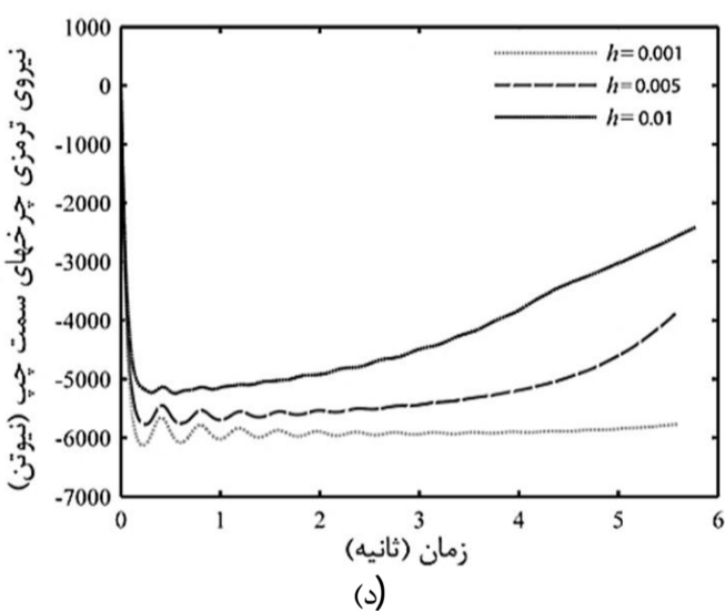
شکل 5 تأثیر زمان پیش‌بین بر مقاومت کنترل‌کننده در چرخ جلو چپ: الف) لغزش، ب) خطای ردیابی لغزش، ج) گشتاور ترمزی، د) نیروی ترمزی
