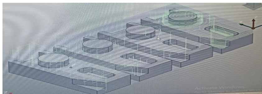
شکل ۱) الف) نمایش نحوه براده‌برداری استراتژی‌های ارائه شده [23] (ب) قطعه سه‌بعدی طراحی شده در کتیا (ج) شبیه‌سازی استراتژی‌های مختلف پرداخت مورداستفاده برای ساخت قطعه موردنظر
