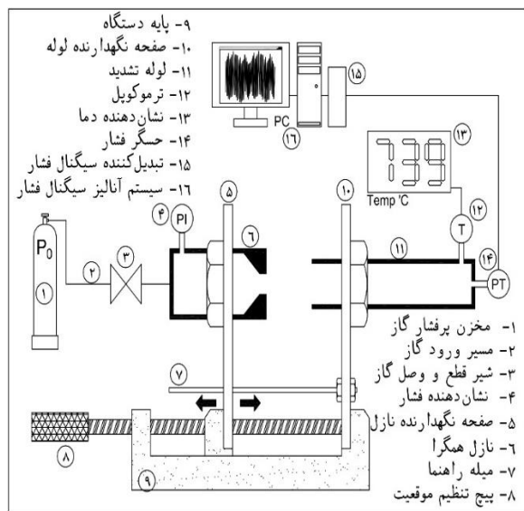
شکل ۴) طرح‌واره نمونه آزمایشگاهی جهت آزمون تجربی
