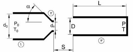
① مسیر ورود گاز ② نازل همگرا ③ لوله تشدید P_0 فشار گاز ورودی به نازل T_0 دمای گاز ورودی به نازل T دمای انتهایی لوله S فاصله بین خروجی نازل و ورودی لوله d_0 قطر ورودی نازل d_n قطر خروجی نازل \alpha زاویه همگرایی نازل D قطر داخلی لوله L طول لوله
