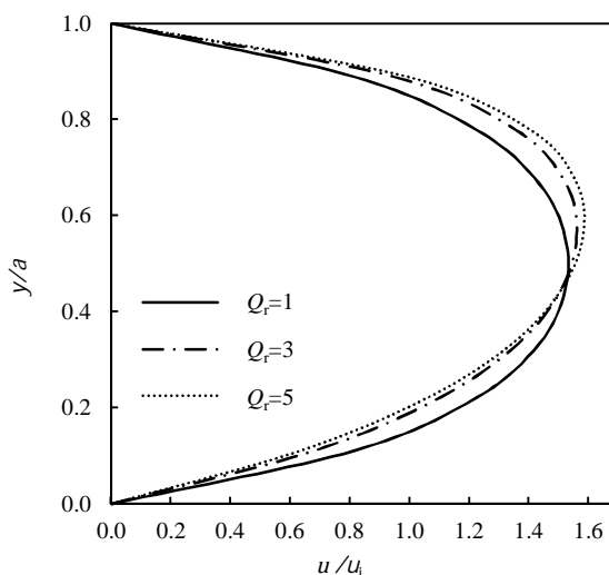
شکل 10 پروفیل سرعت بی بعد در مقطع x/D_n = 50 برای مقادیر مختلف Q_r
