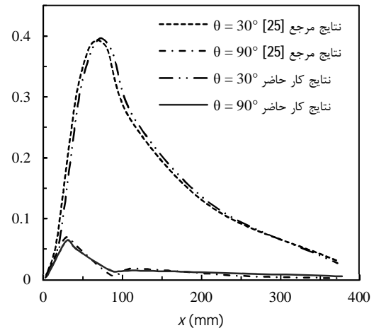
شکل 4 مقایسه شدت بیشینه جریان ثانویه با نتایج عددی ایچیمیا و ماتسوشیما [25] برای سیال تک فاز در Re = 100 ، Ri = 2.2
