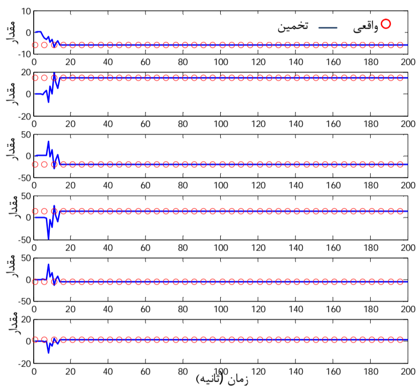
شکل 10 همگرایی ضرایب چندجمله‌ای بدون بعد \gamma(\xi) (خط) به مقدار واقعی (دایره)
