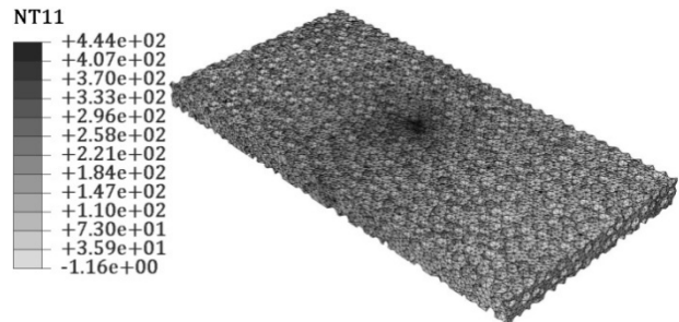
شکل ۱۳ کانتور توزیع دمایی، قدرت لیزر ۱۰۰W، سرعت ۰.۳mm/s، قطر اشعه لیزر ۱/۵mm و تعداد پاس ۱ پاس، زاویه خمش ۰/۸۸۲ درجه
