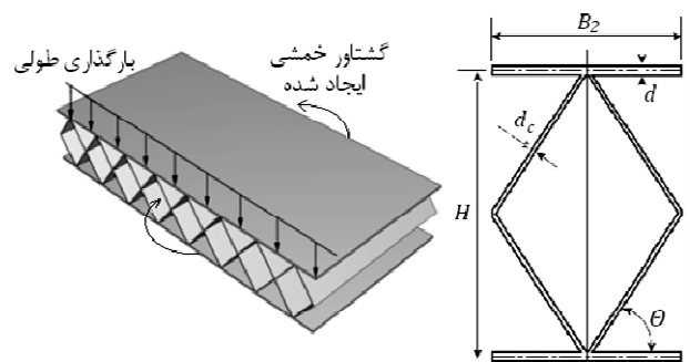
شکل ۱ پانل با n=2 تحت بارگذاری طولی و متغیرهای طراحی
