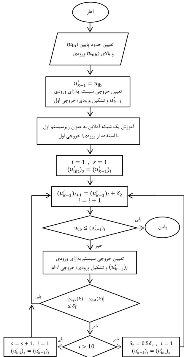
شکل 1 فلوجارت گام نخست الگوریتم پیشنهادی
