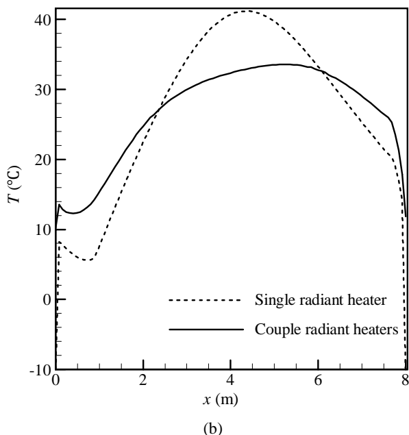
Fig. 9 Temperature distribution of floor of hall for (a) 5 air changes per hours, (b) 10 air changes per hours شکل 9 توزیع دمای کف سالن (الف) تعداد دفعات تعویض هوای 5 بار در ساعت، (ب) تعداد دفعات تعویض هوای 10 بار در ساعت
