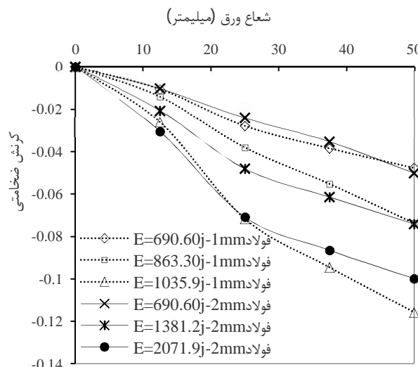
شکل 9 توزیع کرنش ضحامت \epsilon_{\theta} برحسب تغییرات فاصله شعاعی برای ورق‌های فولاد 13 با ضخامت‌های مختلف و بانرژی اعمال شده متفاوت
