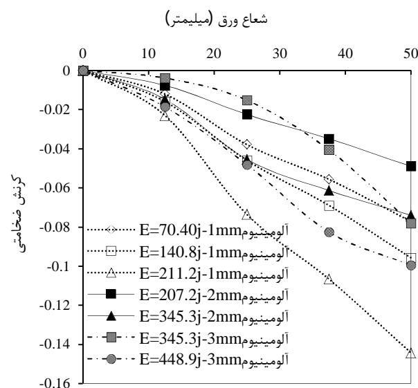
شکل 10 توزیع کرنش ضحامت \epsilon_{\theta} برحسب تغییرات فاصله شعاعی برای ورق‌های آلومینیوم 1100 با ضخامت‌های مختلف و بانرژی اعمال شده متفاوت
