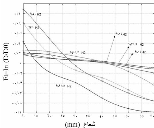
نمودار ۴ تغییرات کرنش ضخامتی به شعاع برای درصدهای مختلف هیدروژن
