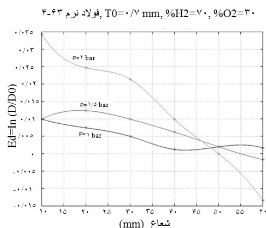
نمودار ۶ تغییرات کرنش ضخامتی نسبت به شعاع
