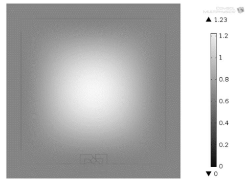
شکل 4 جابه‌جایی دیافراگم تحت فشار 100 کیلوپاسکال (بر حسب میکرومتر)
