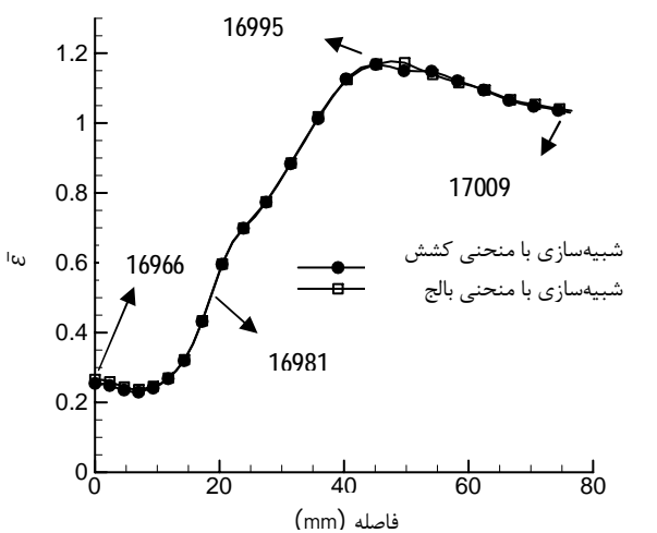
شکل 25 کرنش معادل در امتداد مسیر از گره 16966 تا 17009 در زمان t=36s
