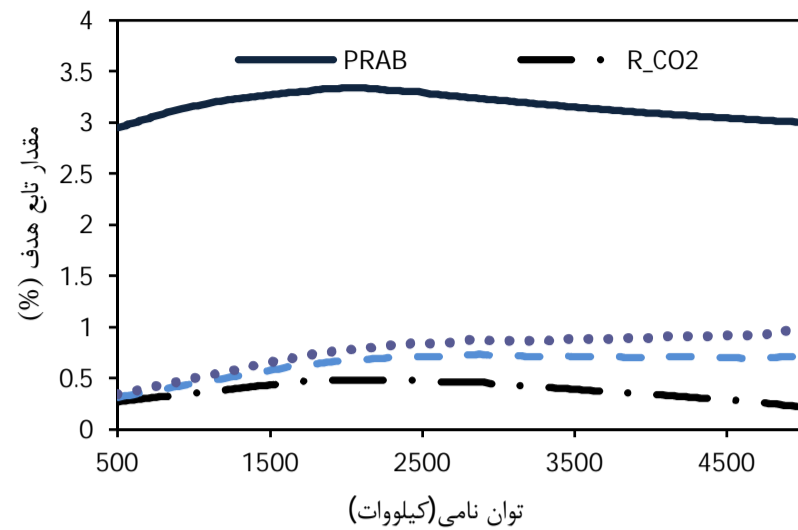
شکل 5 تغییرات توابع هدف بر حسب توان نامی
