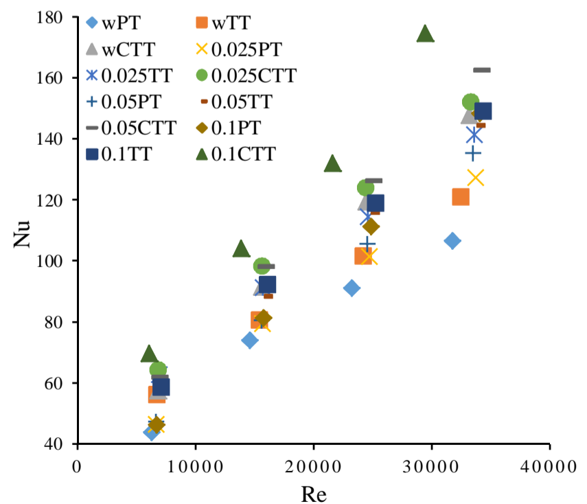
شکل 12 نمودار کلی عدد ناسلت بر حسب عدد رینولدز در دمایی 70 درجه سانتیگراد
