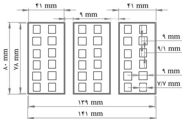
شکل 3 چیدمان تراشه‌ها در هر یک از فازهای تجهیز SKIM606GD066HD و نحوه
