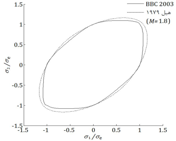
شکل 13 سطح تسلیم پیش‌بینی شده برای آلومینیوم AA5182-O
