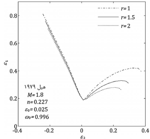
شکل 19 اثر ضریب ناهمسانگردی بر FLD براساس مدل MK و معیار هیل 1979
