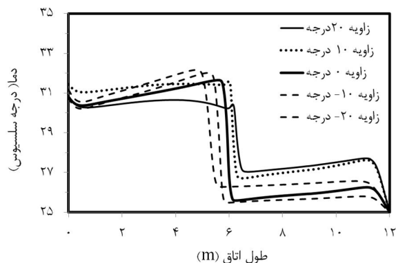
شکل 9 توزیع دما در فضای نمونه بر اثر تغییرات زاویه
