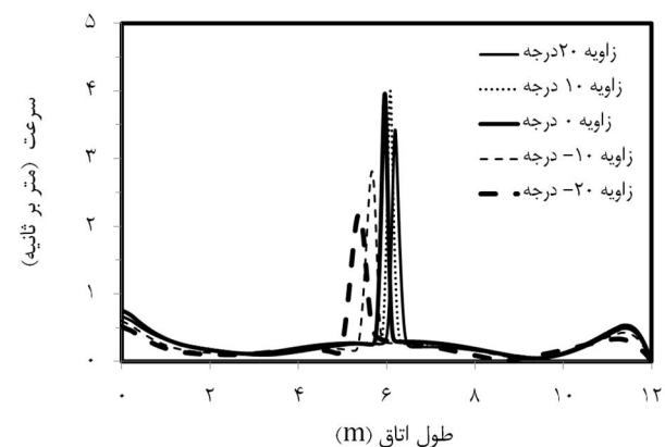
شکل 10 اثرات تغییر زاویه پاشش جت دستگاه پرده هوایی بر توزیع سرعت
