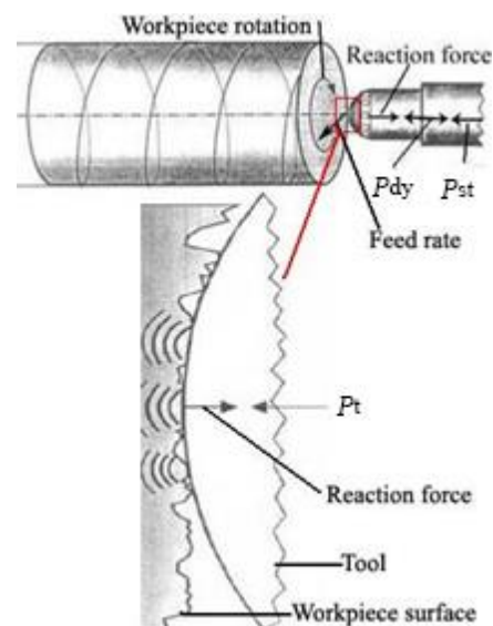
Fig. 2 Schematic representation of UPT tool on the work piece surface شکل 2 نمایش شماتیک ابزار UPT بر روی سطح قطعه کار
