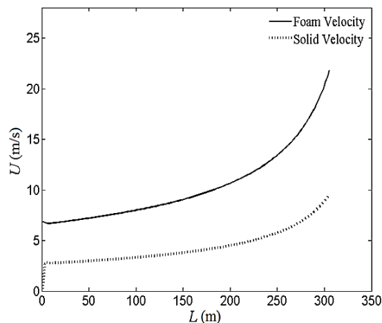
Fig. 7 shows foam cuttings velocity along the well شکل 7 سرعت فوم و کنده‌ها در طول چاه
