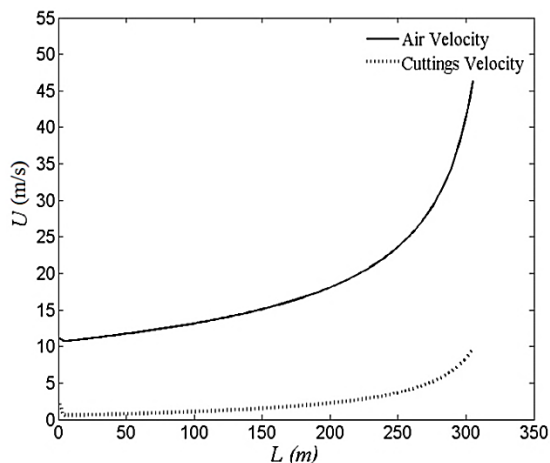
Fig. 8 shows air and cuttings vel L(m) ong the well شکل 8 سرعت هوا و کنده‌ها در طول چاه
