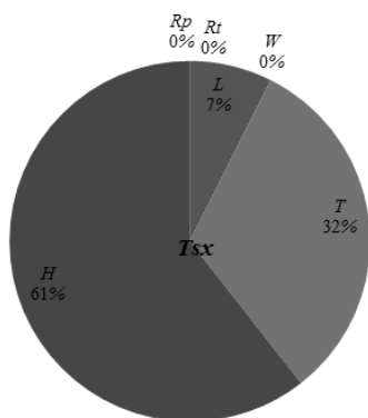
a) Critical time of sliding along the x-axis (الف) زمان بحرانی لغزش در راستای محور x
