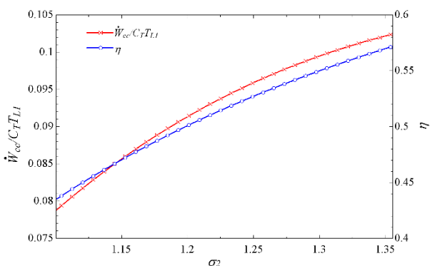
Fig. 4 Variations dimensionless total power and efficiency versus dimensionless variable \sigma_2 شکل 4 رفتار توان کل بی‌بعد و بازده با تغییر متغیر بی‌بعد \sigma_2
