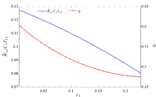
Fig.7 Variations dimensionless total power and efficiency versus r_3 شکل 7 تغییرات توان کل بی‌بعد و بازده نسبت به r_3
