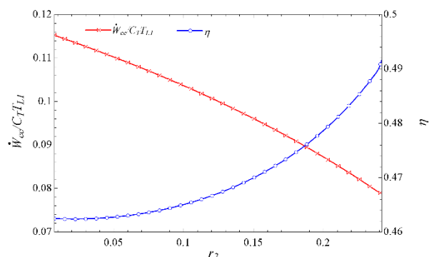
Fig.6 Variations dimensionless total power and efficiency versus r_2 شکل 6 تغییرات توان کل بی‌بعد و بازده نسبت به r_2
