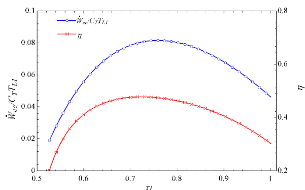
Fig.9 Efficiency and dimensionless total power versus \tau_1 شکل 9 تغییرات توان کل بی‌بعد و بازده نسبت به \tau_1
