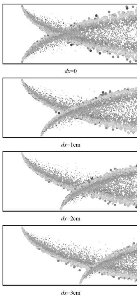
Fig. 7 the droplets sprayed from two injectors in a duct in various distances of between the injectors ( \theta_1=\theta_2=70^\circ , \varphi=180^\circ , \alpha=15^\circ , t=100\text{ms} ) شکل 7 قطرات پاشش شده از دو اسپری در مجرا در فواصل مختلف دو انژکتور ( \theta_1=\theta_2=70^\circ , \varphi=180^\circ , \alpha=15^\circ , t=100\text{ms} )
