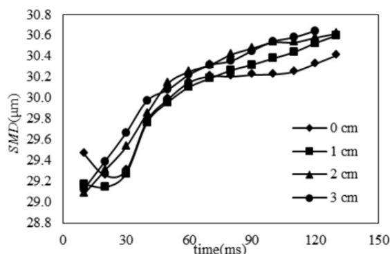
Fig. 8 The SMD of the droplets based on the time in distances of between the injectors ( \theta_1=\theta_2=70^\circ , \varphi=180^\circ , \alpha=15^\circ ) شکل 8 قطر متوسط قطرات بر حسب زمان در موقعیت‌های طولی مختلف انژکتور دوم ( \theta_1=\theta_2=70^\circ , \varphi=180^\circ , \alpha=15^\circ )
