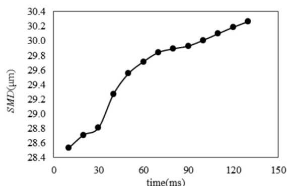
Fig. 6 The SMD of the droplets based on the time in single injector ( \theta_1=70^\circ , x_1=30\text{mm} , \alpha=15^\circ ) شکل 6 قطر متوسط قطرات بر حسب زمان در تک انژکتور، ( \theta_1=70^\circ , x_1=30\text{mm} , \alpha=15^\circ )
