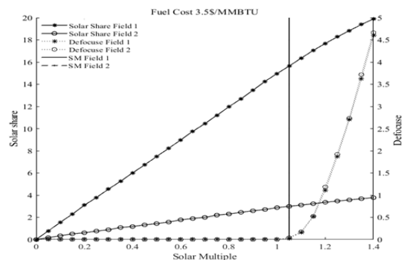
نمودار ۸ اثر تغییرات ضریب مساحت میدان خورشیدی برای هر دو میدان خورشیدی برای بهترین مدل روی سهم انرژی خورشیدی و میزان ناکانونی براساس راه اول (قیمت گاز طبیعی ۳/۵ دلار به ازای هر میلیون بی‌تی‌یو)
