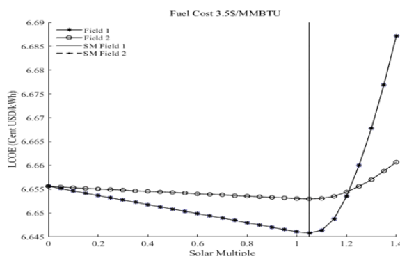
نمودار ۹ اثر تغییرات ضریب مساحت میدان خورشیدی برای هر دو میدان خورشیدی برای بهترین مدل روی LCOE براساس راه اول (قیمت گاز طبیعی ۳/۵ دلار به ازای هر میلیون بی‌تی‌یو)
