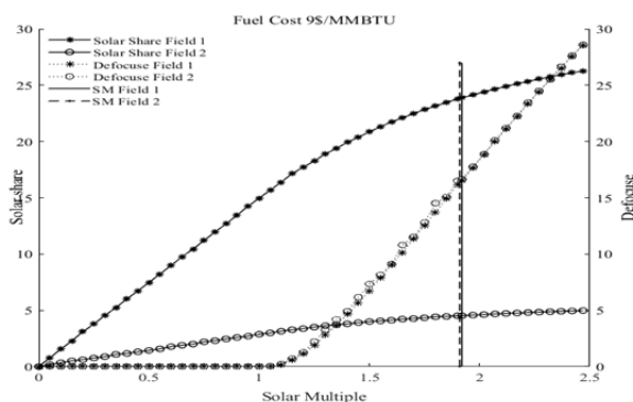
نمودار ۱۰ اثر تغییرات ضریب مساحت میدان خورشیدی برای هر دو میدان خورشیدی برای بهترین مدل روی سهم انرژی خورشیدی و میزان ناکانونی براساس راه اول (قیمت گاز طبیعی ۹ دلار به ازای هر میلیون بی‌تی‌یو)
