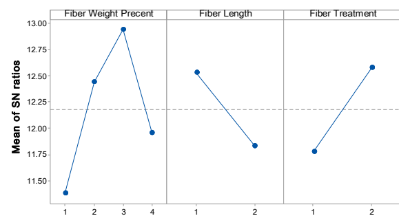
نمودار ۴) نمودار سیگنال به نویز برای مدول الاستیسیته کششی کامپوزیت
