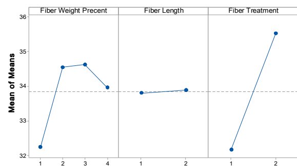
نمودار ۱) نمودار میانگین‌های استحکام کششی کامپوزیت
