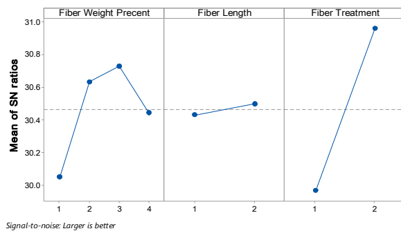
نمودار ۲) نمودار سیگنال به نویز برای استحکام کششی کامپوزیت
