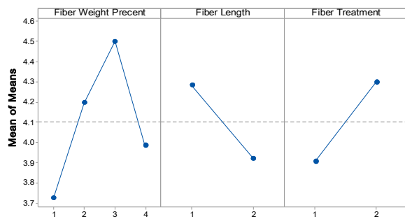
نمودار ۳) نمودار میانگین‌های مدول الاستیسیته کششی کامپوزیت
