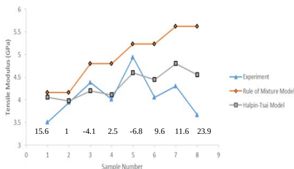
نمودار ۱۲) نتایج مدل‌های میکرومکانیک برای مدول الاستیسیته کششی نمونه‌ها و درصد خطای مدل اصلاح‌شده هالپین-تسای نسبت به نتایج تجربی
