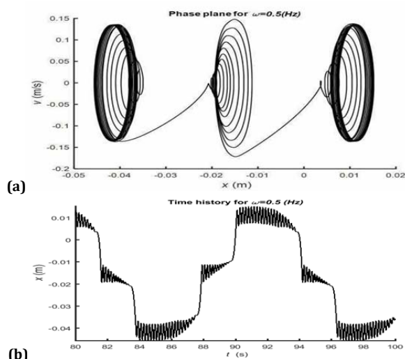
نمودار ۳) پاسخ ارتعاشات آزاد نوسانگر آلیاژ حافظه‌دار در پژوهش انجام شده توسط ماچادو و همکاران
