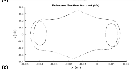
نمودار ۷ صفحه فاز، محتوای فرکانسی و نگاشت پوانکاره مربوط به نوسانگر آلیاژ حافظه‌دار در \omega=4\text{Hz} . (a) صفحه فاز (b) محتوای فرکانسی (c) نگاشت پوانکاره مربوط به نوسانگر آلیاژ حافظه‌دار
