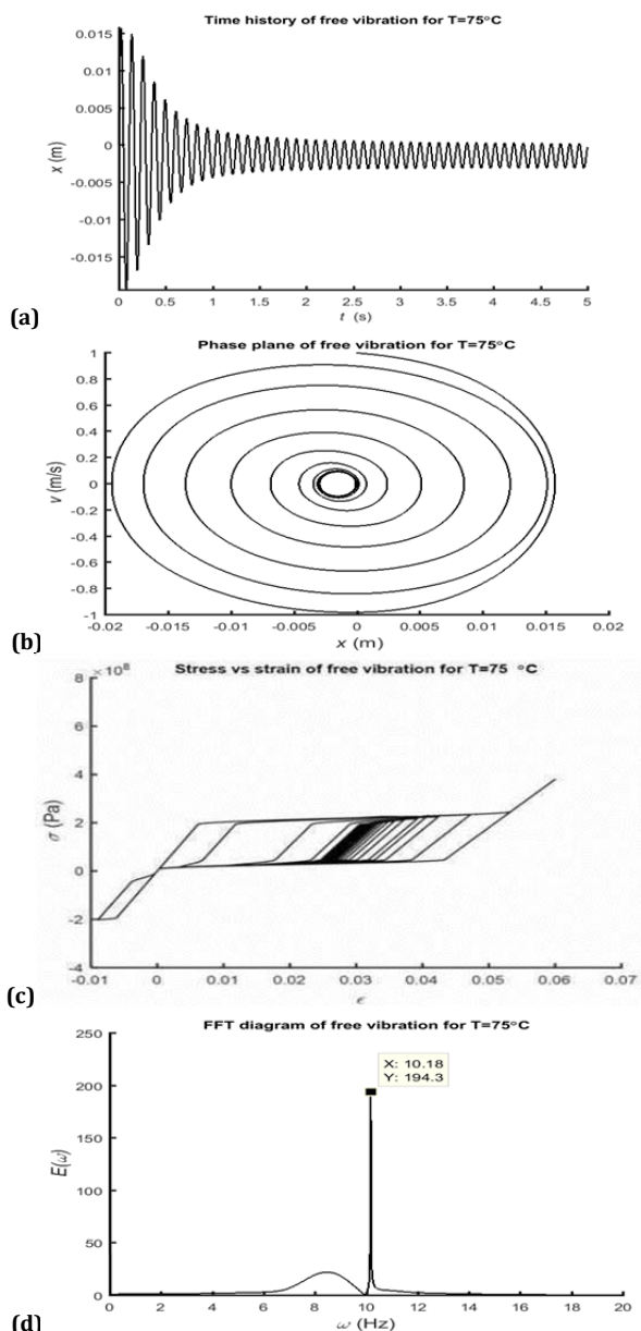
نمودار ۲ پاسخ ارتعاشات آزاد نوسانگر آلیاژ حافظه‌دار، (a) تاریخچه زمانی (b) صفحه فاز (c) تنش بر حسب کرنش (d) نمودار محتوای فرکانسی
