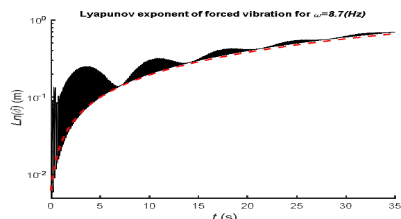
نمودار ۱۰) نمای لیاپانوف مربوط به نوسانگر آلیاژ حافظه‌دار در \omega=8/7\text{Hz}
