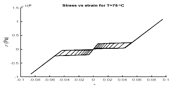
نمودار ۱ اثر سوپرالاستیک آلیاژ حافظه‌دار با احتساب تقارن در کشش و فشار
