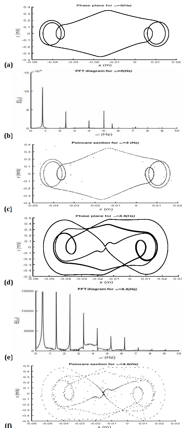
نمودار ۸) صفحه فاز، محتوای فرکانسی و نداشت پوانکاره مربوط به نوسانگر آلیاژ حافظه‌دار در \omega = 5 Hz و \omega = 8.6 Hz. (a) صفحه فاز (b) محتوای فرکانسی (c) نداشت پوانکاره مربوط به نوسانگر آلیاژ حافظه‌دار در \omega = 5 Hz (d) صفحه فاز (e) محتوای فرکانسی (f) نداشت پوانکاره مربوط به نوسانگر آلیاژ حافظه‌دار در \omega = 8.6 Hz
