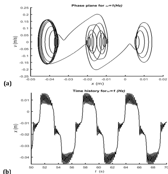
نمودار ۵) صفحه فاز و پاسخ زمانی نوسانگر آلیاژ حافظه‌دار در \omega=1\text{Hz} (a) صفحه فاز (b) پاسخ زمانی نوسانگر آلیاژ حافظه‌دار
