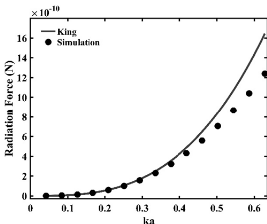
نمودار ۶) مقایسه نیروی تابشی آکوستیک شبیه‌سازی شده با تئوری کینگ بر حسب افزایش شعاع ذره
