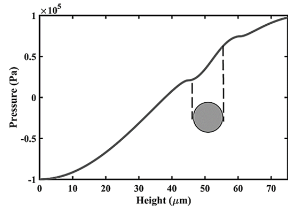
نمودار ۱) توزیع فشار در راستای خط قائم گذرنده از ذره کروی در میکروکانال
